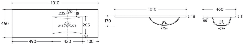
Cerámico Cuadrado 101x46cm desplazado derecha (40+60)
