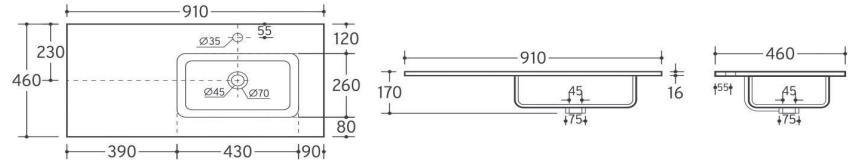
Cerámico Perfect 91x46cm desplazado derecha (30+60)
