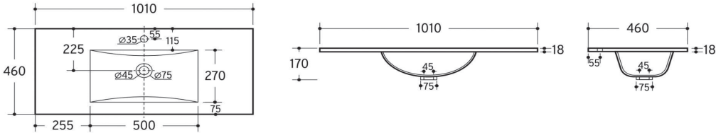
Cerámico Cuadrado 101x46cm
