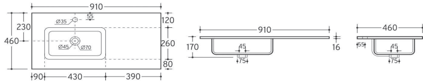
Cerámico Perfect 91x46cm desplazado izquierda (60+30)
