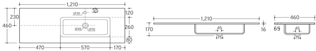
Cerámico Perfect 121x46cm desplazado derecha (30+90)
