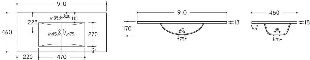
Cerámico Cuadrado 91x46cm
