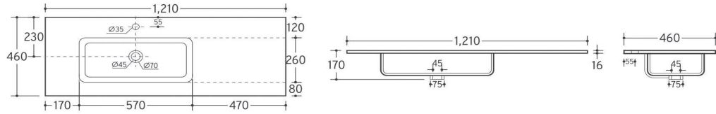
Cerámico Perfect 121x46cm desplazado izquierda (90+30)
