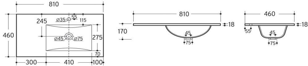
Cerámico Cuadrado 81x46cm desplazado derecha (20+60)
