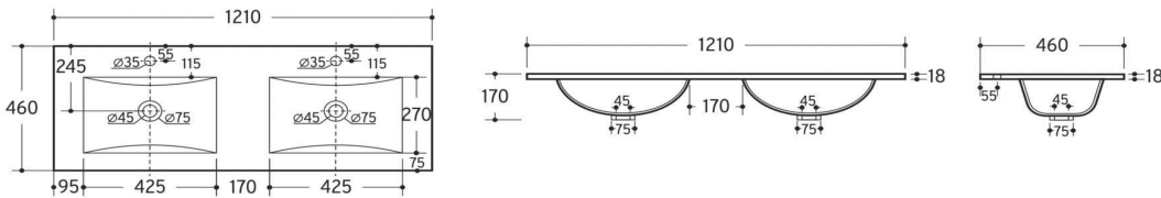
Cerámico Cuadrado 121x46cm 2s
