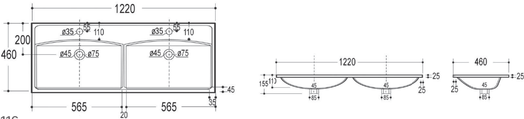
Galaxy 121x46cm 2s
