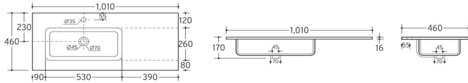
Cerámico Perfect 101x46cm desplazado izquierda (70+30)
