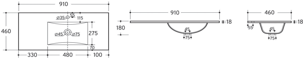
Cerámico Cuadrado 91x46cm desplazado derecha (20+70)
