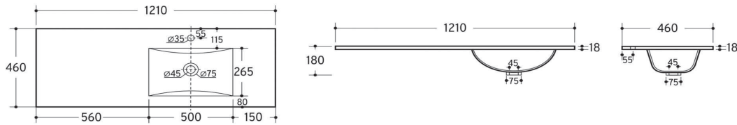
Cerámico Cuadrado 121x46cm desplazado derecha (40+80)
