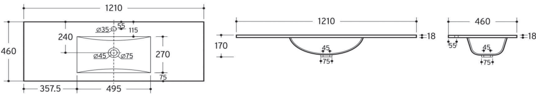
Cerámico Cuadrado 121x46cm 1s
