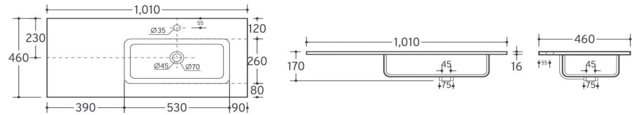
Cerámico Perfect 101x46cm desplazado derecha (30+70)
